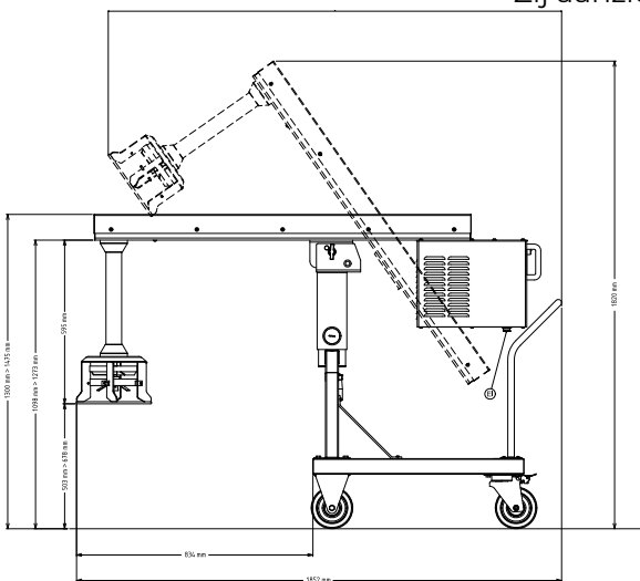
Zij aanzicht
